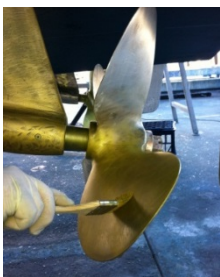
Prima mano di primer
